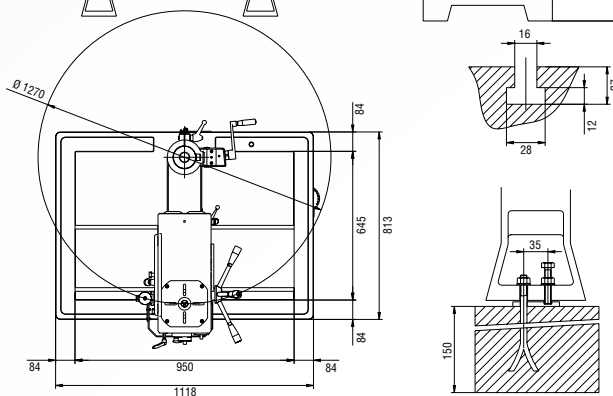
SERIE MSM-MSVM 18-25
