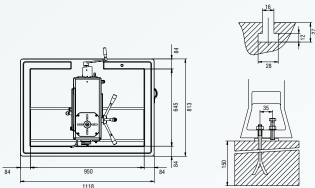
SERIE MS-MSV 18-25-30
