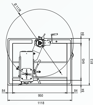
SERIE MSG-MSVG 18-25
