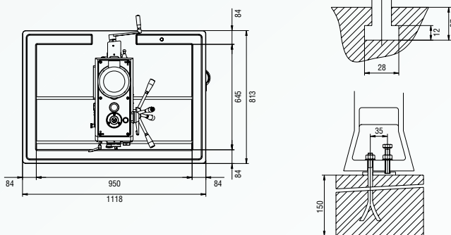
SERIE MSE-MSEA 25-30
